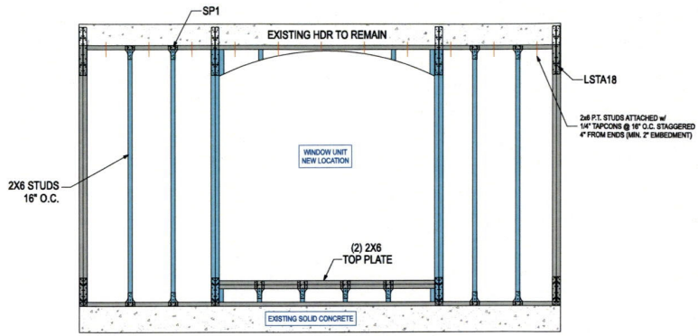
A NEW WINDOW OPENING SCALE: N.T.S.
