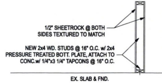
KNEE WALL DETAIL SCALE: (N.T.S.)
