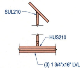
D 2x10 SUPPORT CONNECTION DETAIL SCALE: N.T.S.
