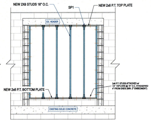
B NEW INFILL SCALE: N.T.S.
