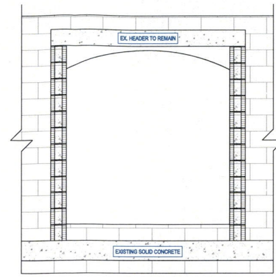
EX. WINDOW OPENING SCALE: N.T.S.
