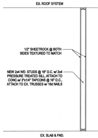
NON-LOAD BEARING WALL DETAIL SCALE: (N.T.S.)
