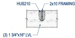
C 2x10 TO LVL CONNECTION DETAIL SCALE: N.T.S.
