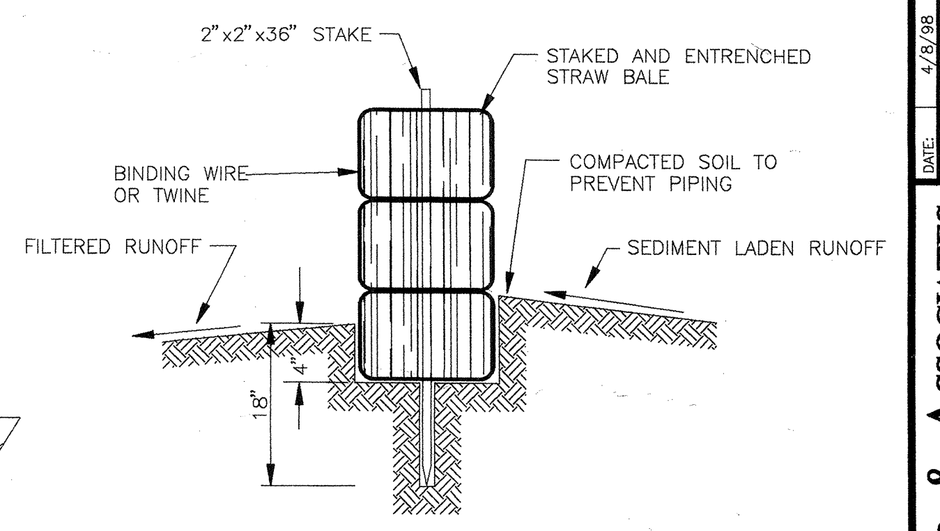
SECTION A-A
