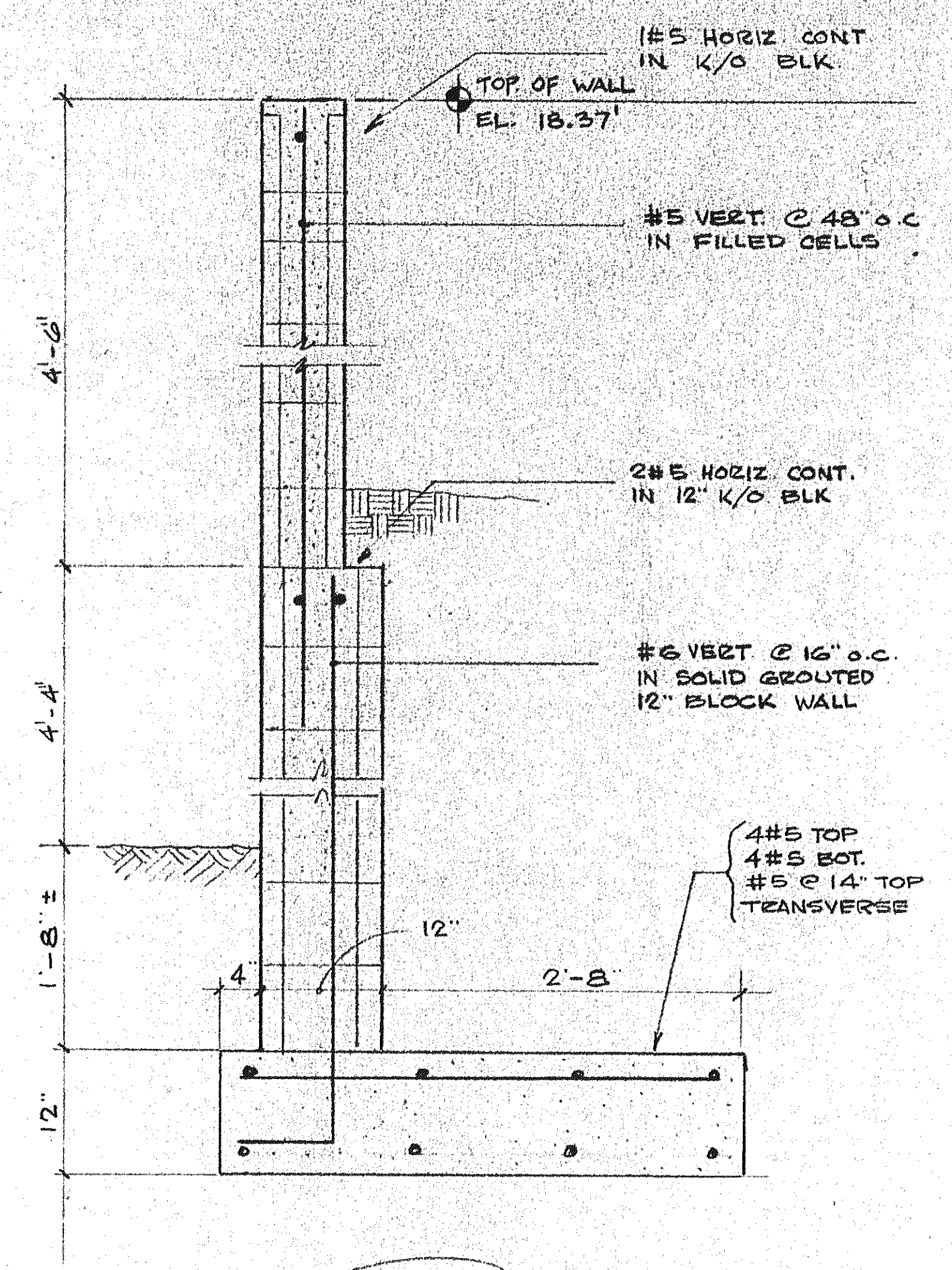
SECTION B SCALE: 1" = 1'-0"
