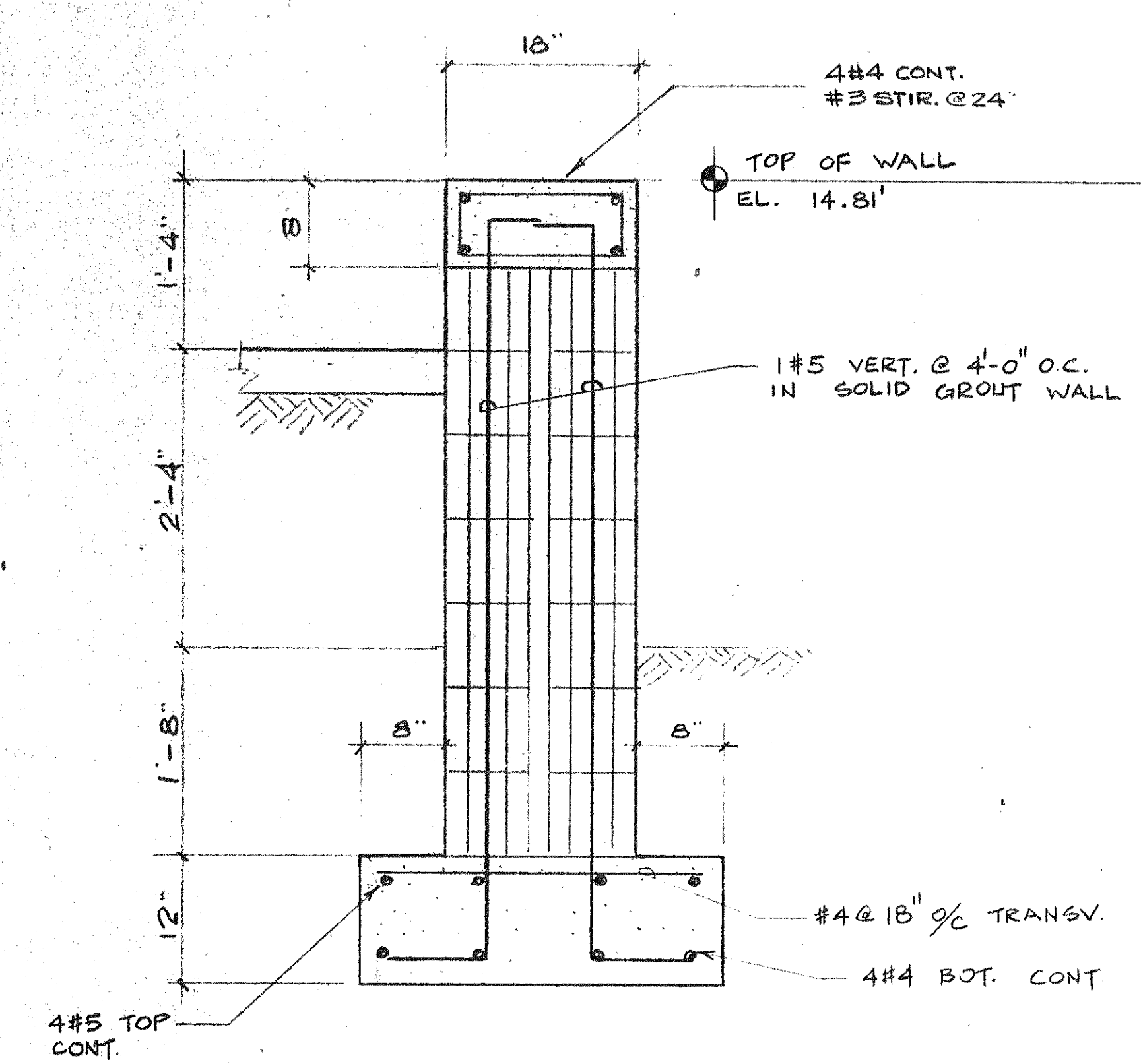
SECTION C SCALE: 1" = 1'-0"
