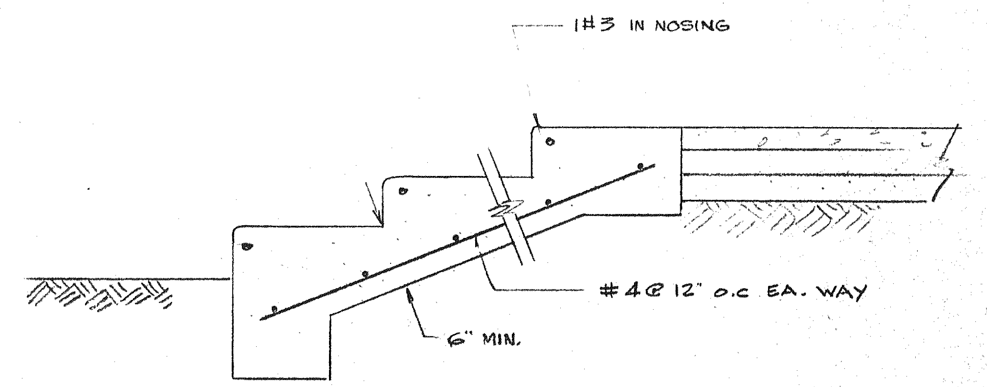
SECTION D SCALE: 1" = 1'-0"
